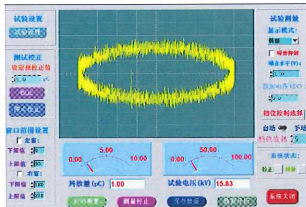
A2: 试验回路1红芯在15kV下局部放电试验图形
