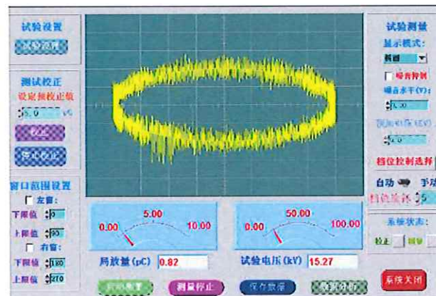
A4: 试验回路1绿芯在15kV下局部放电试验图形
