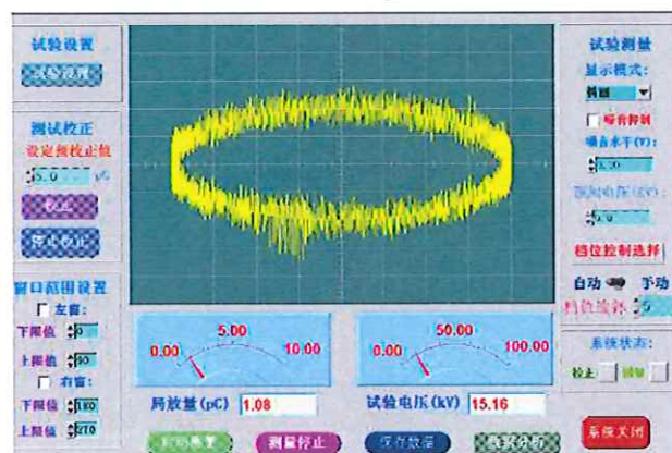
A3: 试验回路1黄芯在15kV下局部放电试验图形
